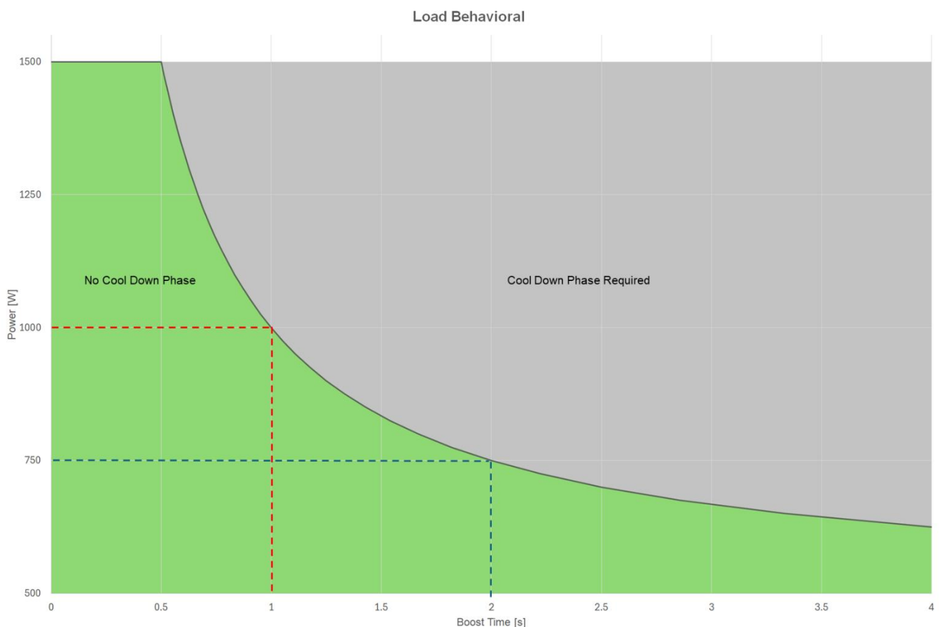
Abbildung –81 : Lastverhalten
