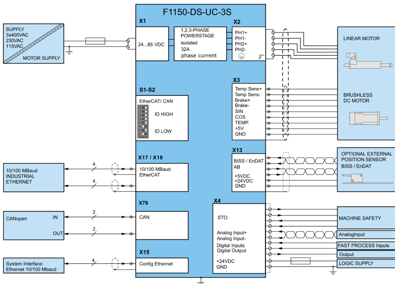
Exemple de système d'asservissement F1150-DS-UC-3S : variateur, moteur et alimentation
