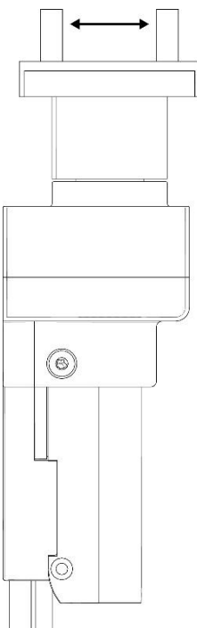
Beispiel 2: vertikale Montage «Greifer oben». Greifen, Platzieren, Montieren, Vereinzeln, Spreizen, Ausrichten sowie Zentrieren von Produkten.
