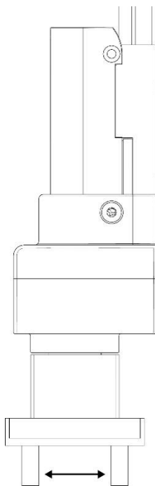
Beispiel 1: vertikale Montage «Greifer unten». Greifen, Ablegen, Montieren, Stapeln, Ausrichten sowie Zentrieren von Produkten.
