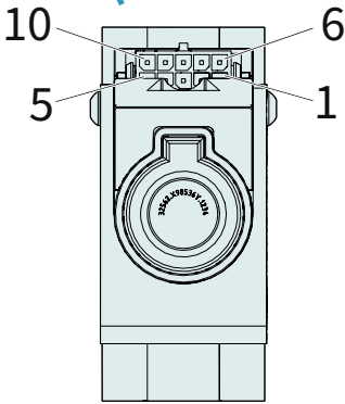
Ansicht: Motorstecker, steckseitig
