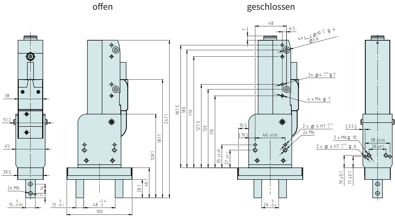
Abmessungen mm
