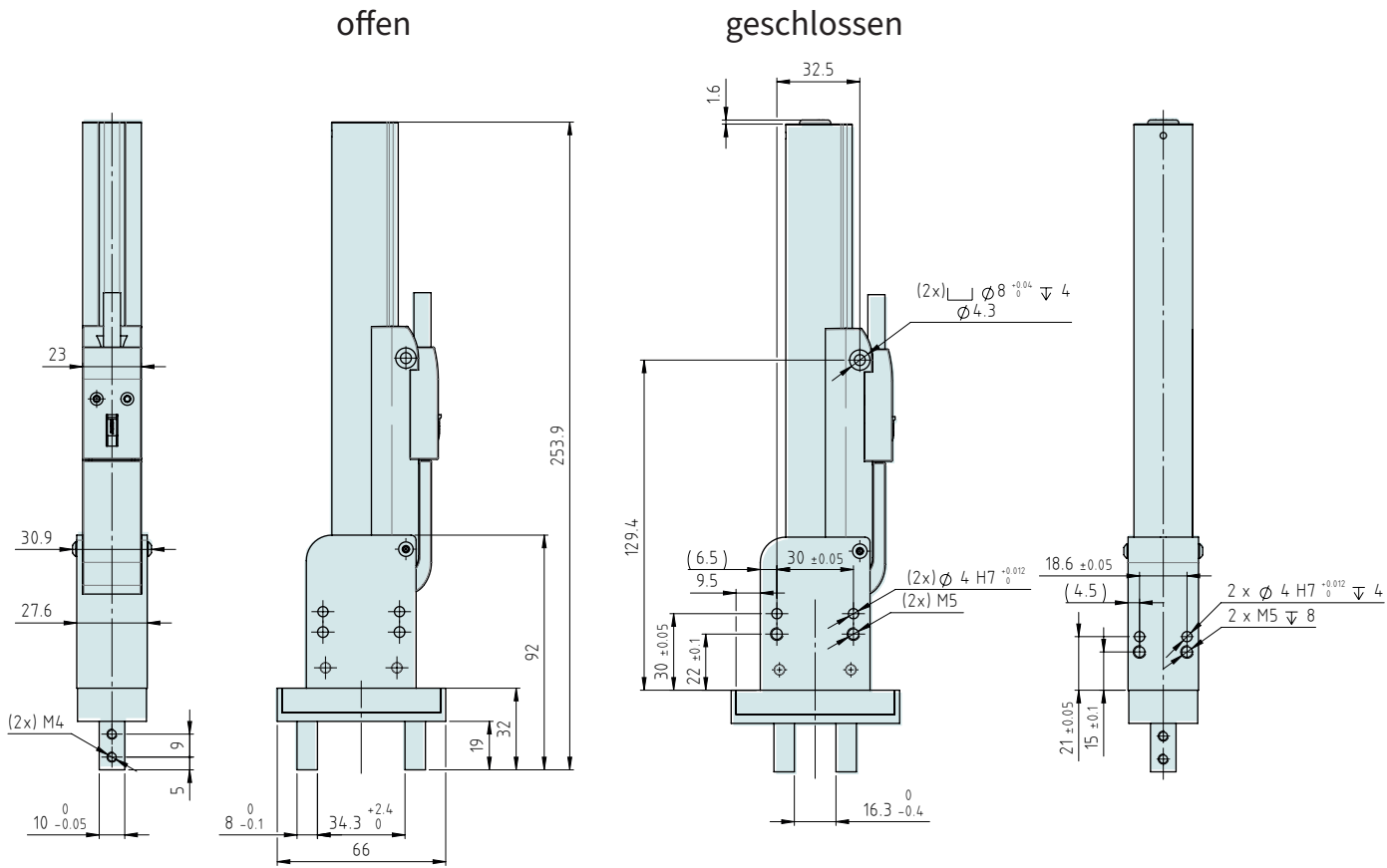
Abmessungen mm
