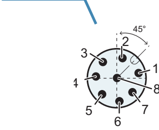
Ansicht: Motorstecker, steckseitig
