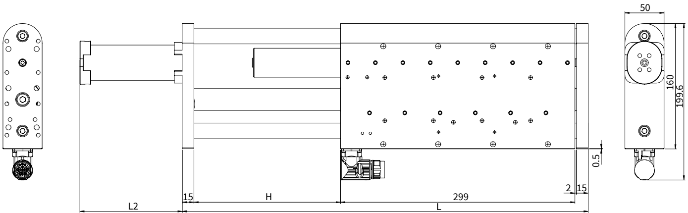
Abmessungen mm
