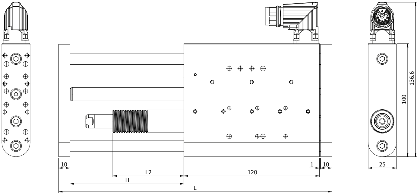
Abmessungen mm
