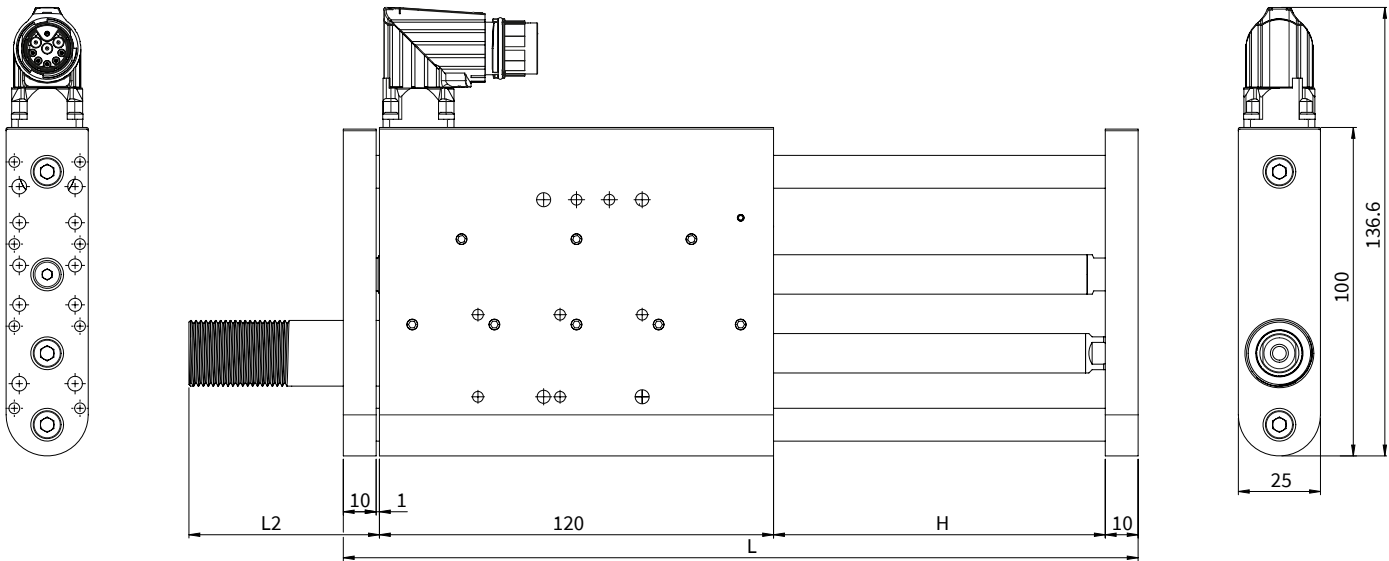
Abmessungen mm
