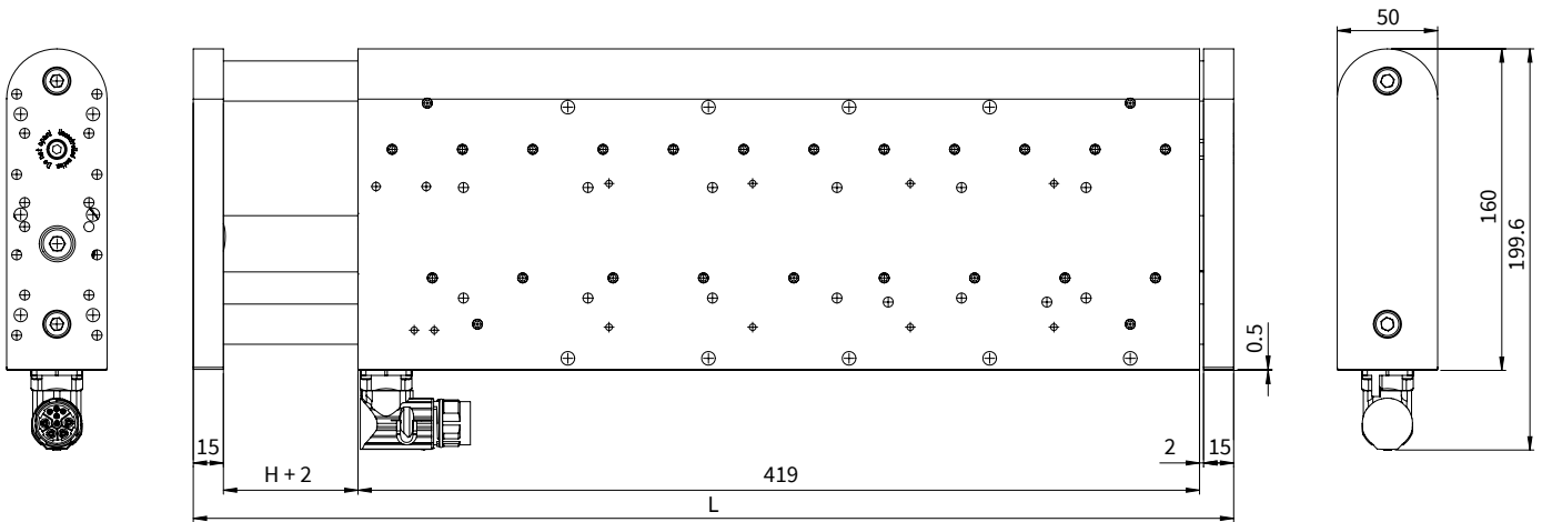
Abmessungen mm
