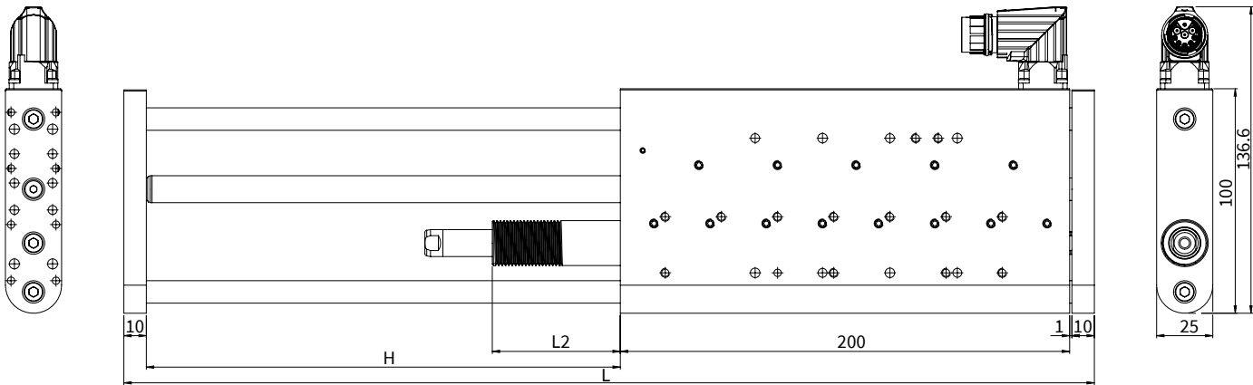
Abmessungen mm
