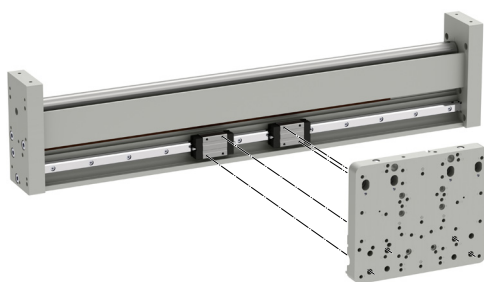
Linearmodul mit einem Carriage Kit
