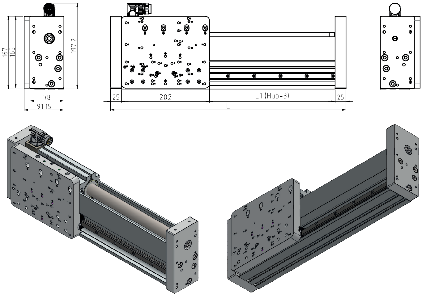
Abmessungen mm
