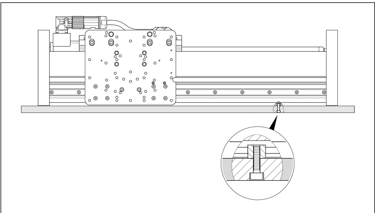
Beispiel 2: Stehende Befestigung unter Verwendung von Nutensteinen von der Unterseite der Modulbasis.
