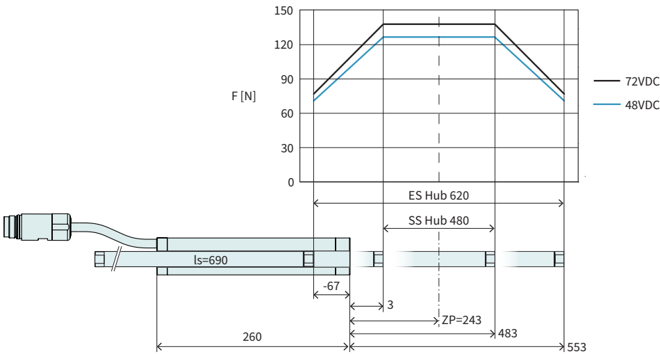
Technische Daten P01-23x160H/480x620-HP-SSCP
