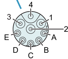
Ansicht: Motorstecker, steckseitig
