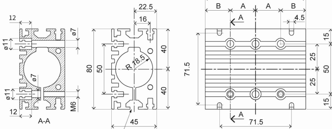
Sliding block M6 (Item-No. 0150-3245)
