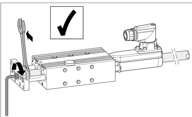
Richtige Montage
