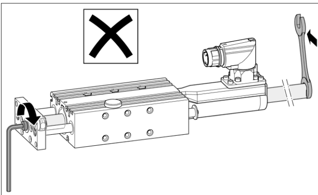
Falsche Montage
